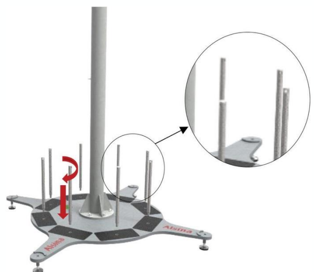
Fig. 7. Fixation des tiges de contrepoids
